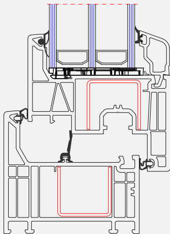
Elegant S76 flächenversetzt vertikal mit runden Glasleisten
