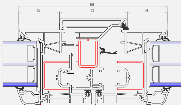
Elegant S76 flächenversetzt horizontal mit runden Glasleisten
